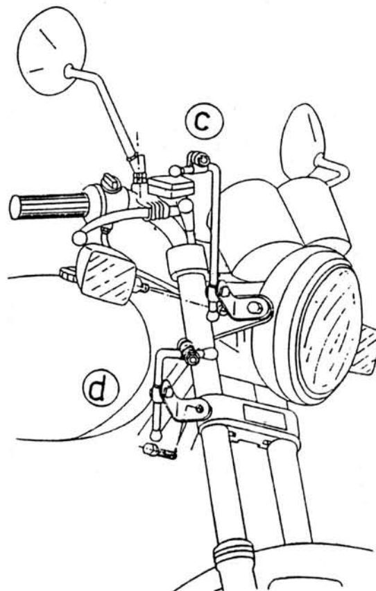
SISTEMA c-d: SUPPORTO FANALE E SUP- PORTO STELO AMMORTIZZATORE a-b SYSTEM: HEAD LAMP AND FORK SUPPORT
