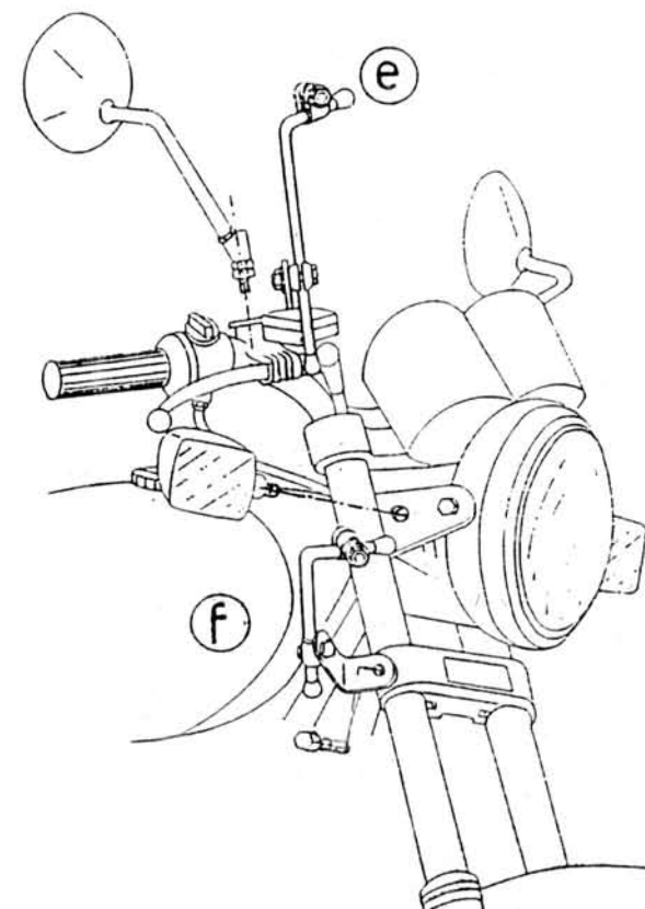
SISTEMA a-b: SUPPORTO SPECCHIETTO E SUPPORTO STELO AMMORTI- ZZATORE a-b SYSTEM: MIRROR AND FORK SUPPORT
