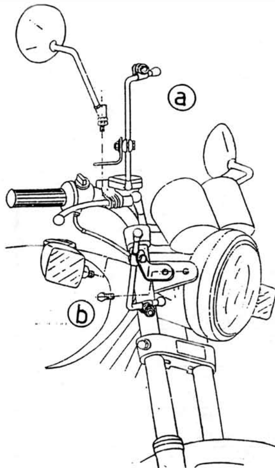
SISTEMA a-b: SUPPORTO SPECCHIETTO E SUPPORTO FANALE a-b SYSTEM: MIRROR AND HEAD LAMP SUPPORT
